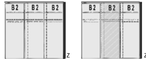
Schwebetürenschränk 2 Mittelwände 6 Einlegeböden 3 Kleiderstangen
